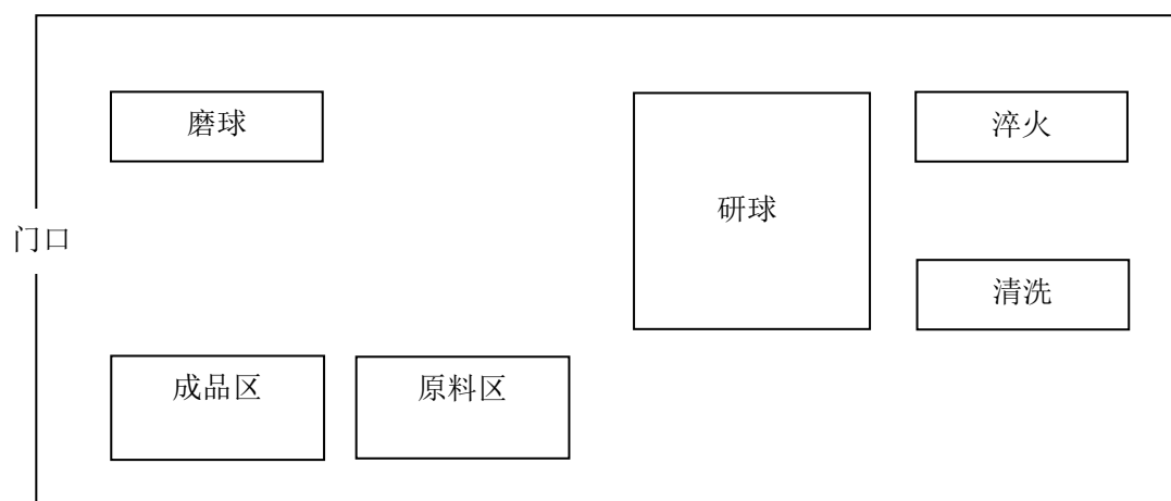
图 2-2 平面布置图
